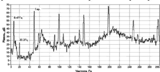
Рис. 2 Прямий спектр вібрації
