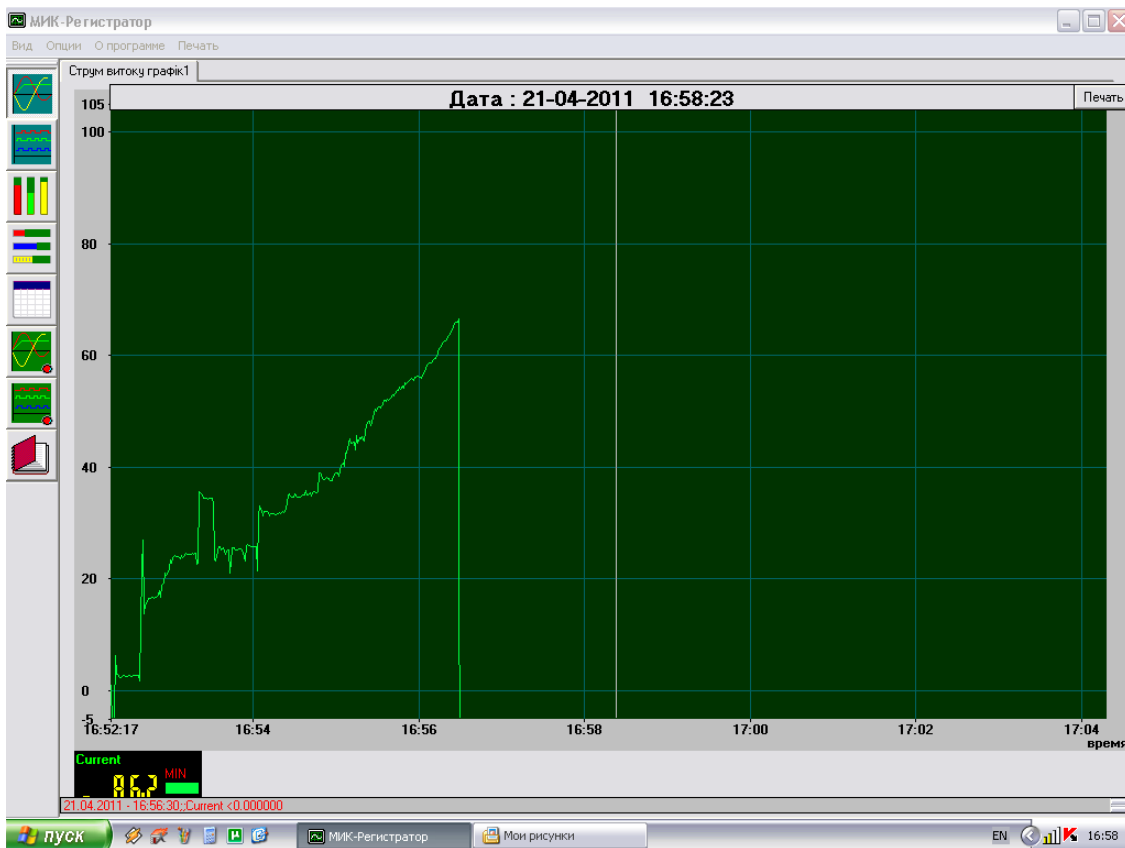
Рис.4. Графік струмів витоку в програмі «МИК-Регистратор»
